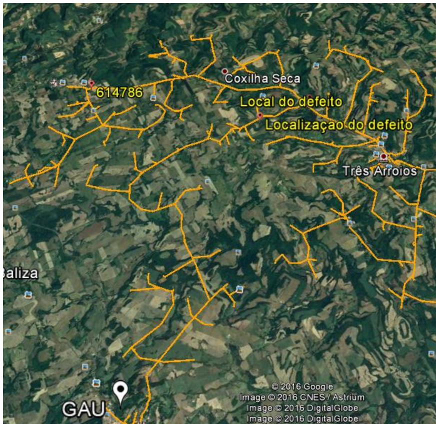
SE Gaurama (GAU) – Unifilar geoeletrico da rede primária de distribuição (alimentadores)
