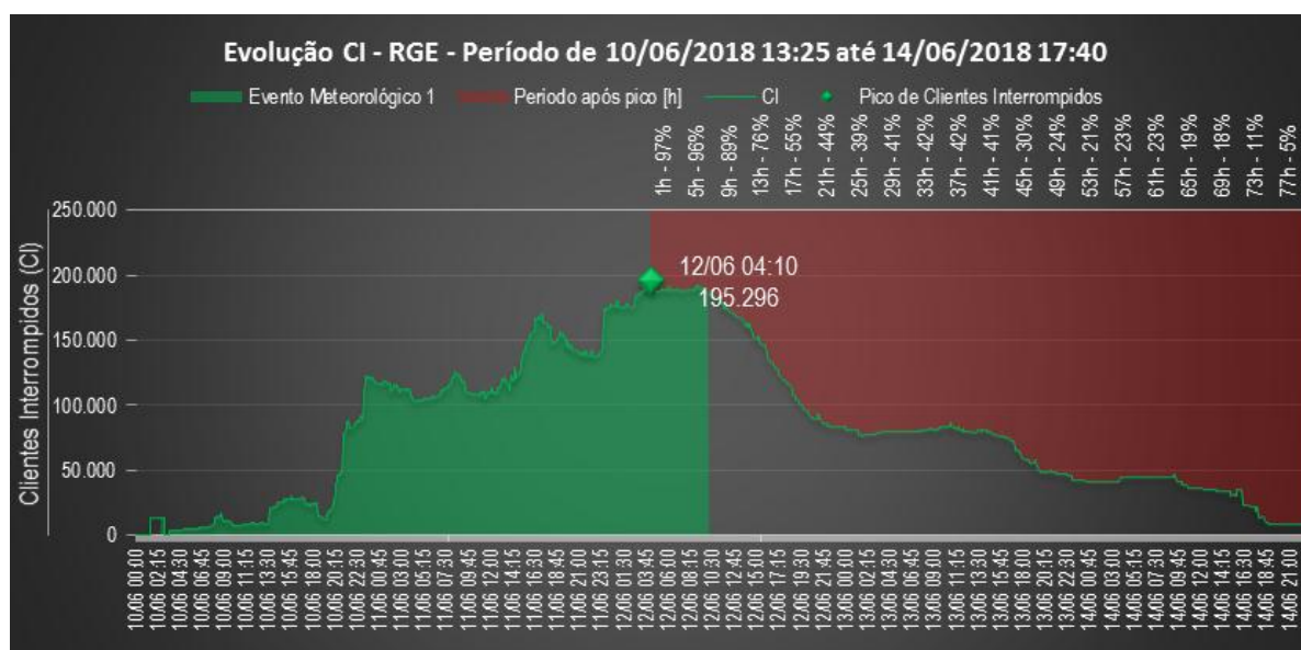
Figura 5 – Quantidade de clientes interrompidos e reestabelecidos no decorrer do evento climatológico.
